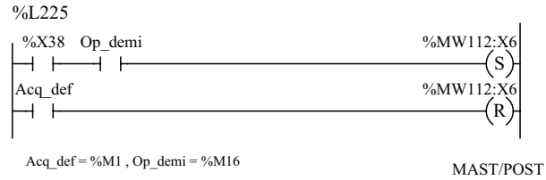
(* Gestion des surveillance de vérin tiroir *)
