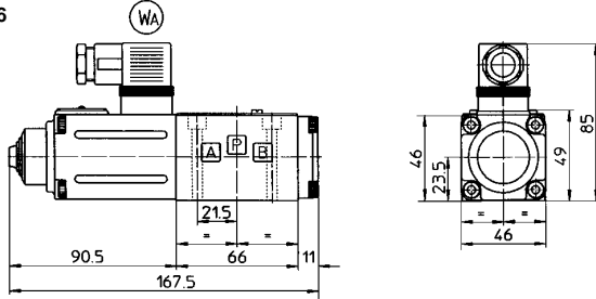
Poids: 1,9 kg
