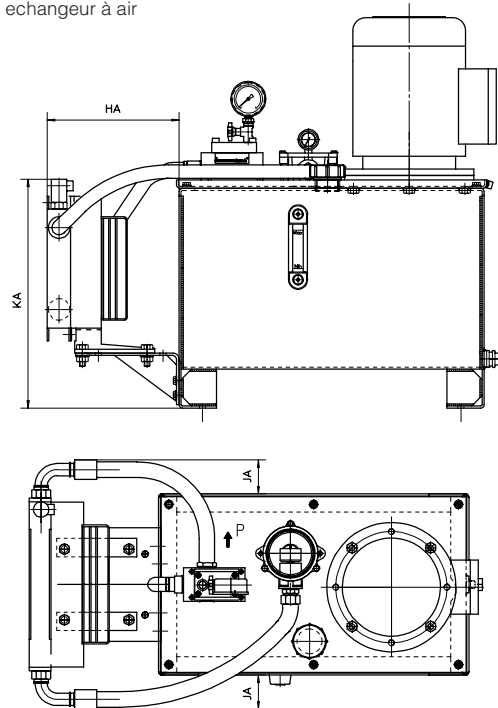
Option /EA Avec échangeur à air
