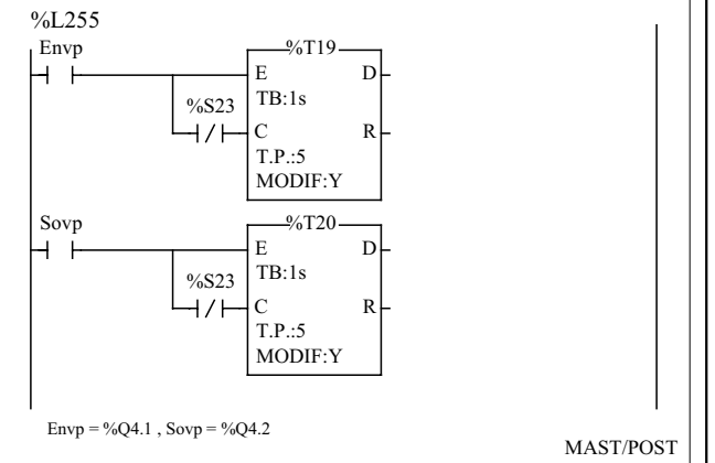
(* Gestion de défaut vérin pousoir *)
