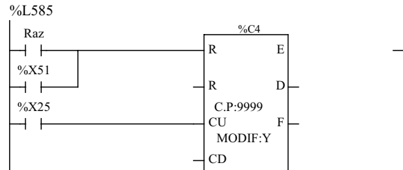
(* Compteur briquette *)
