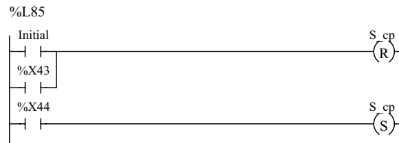
(* Bit de comptage nombre briquette *)
