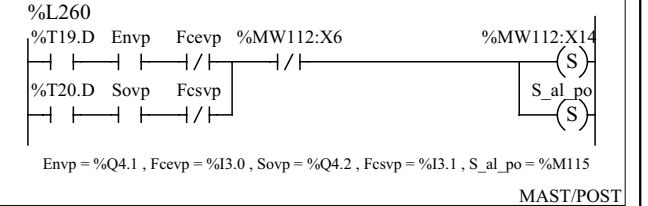
(* Gestion de défaut vérin pousoir *)
