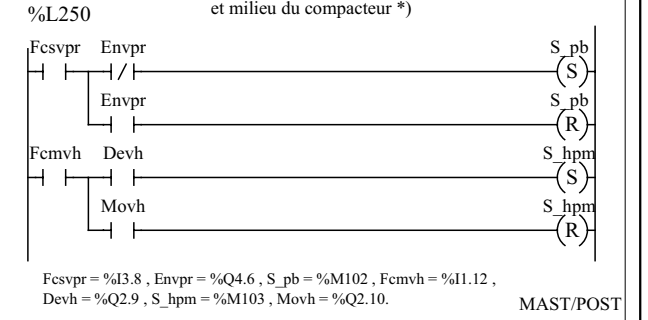
(* Gestion des surveillance de vérin pousoir *)
