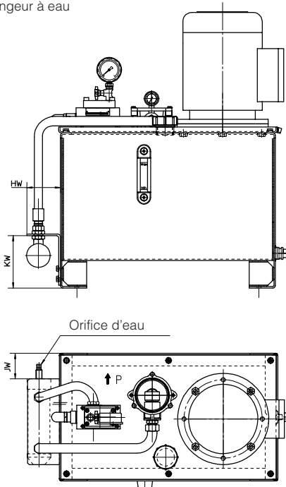
Option /EW Avec échangeur à eau
