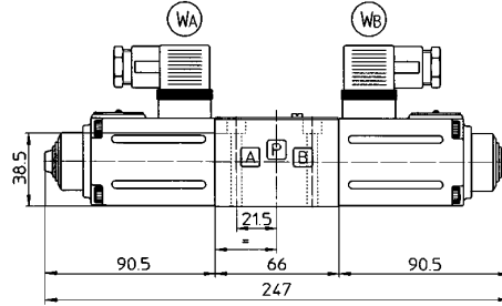
Poids: 2,6 kg
