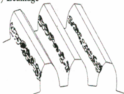
b) Écaillage
