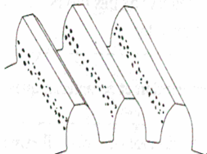
a) Piqûres
